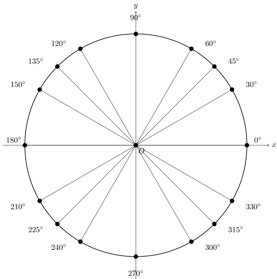
Unit Circle
